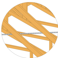
Positionnement des feuilards FP-FPIX sur chevrons avec tendeur de feuillard FMBS au centre
