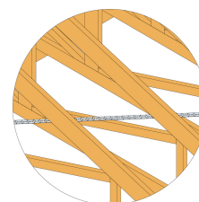
Positionnement des feuillards FP-FPIX sur chevrons avec tendeur de feuillard FMBS au centre
