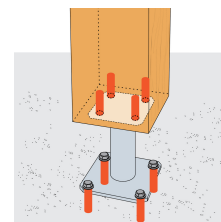
Fixation pied de poteau sur support rigide
