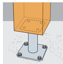
Fixation pied de poteau sur support rigide
